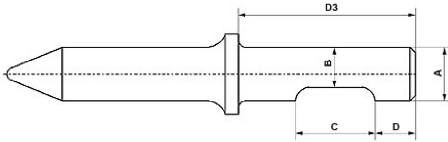
SPIT CU 1 CANAL DE PANA SI GULER
