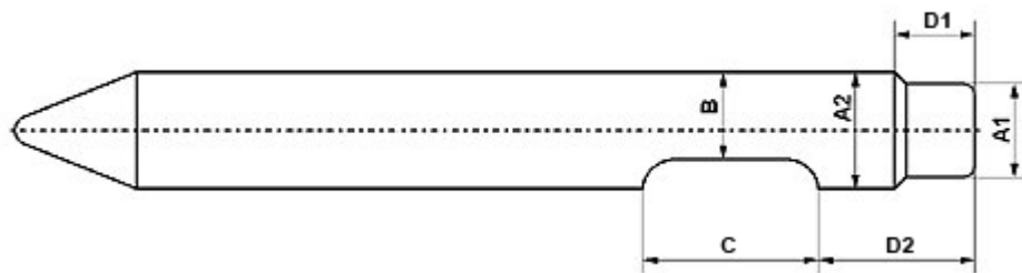
SPIT CU 1 CANAL DE PANA SI CAPAT SUPERIOR INGUST
