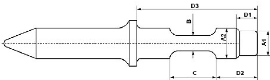
SPIT CU 2 CANALE DE PANA SI GULER
