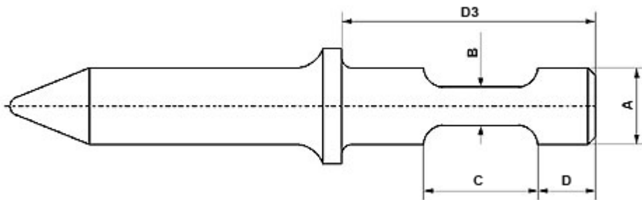
SPIT CU 2 CANALE DE PANA SI GULER
