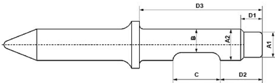
SPIT CU 1 CANAL DE PANA ,GULER SI CAPAT SUPERIOR INGUST
